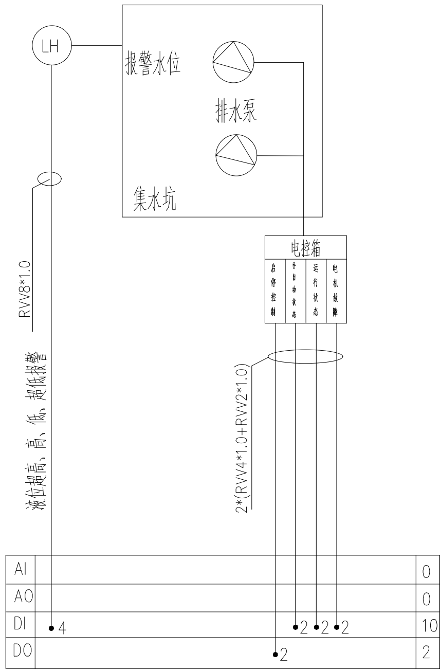
排污泵控制原理图
